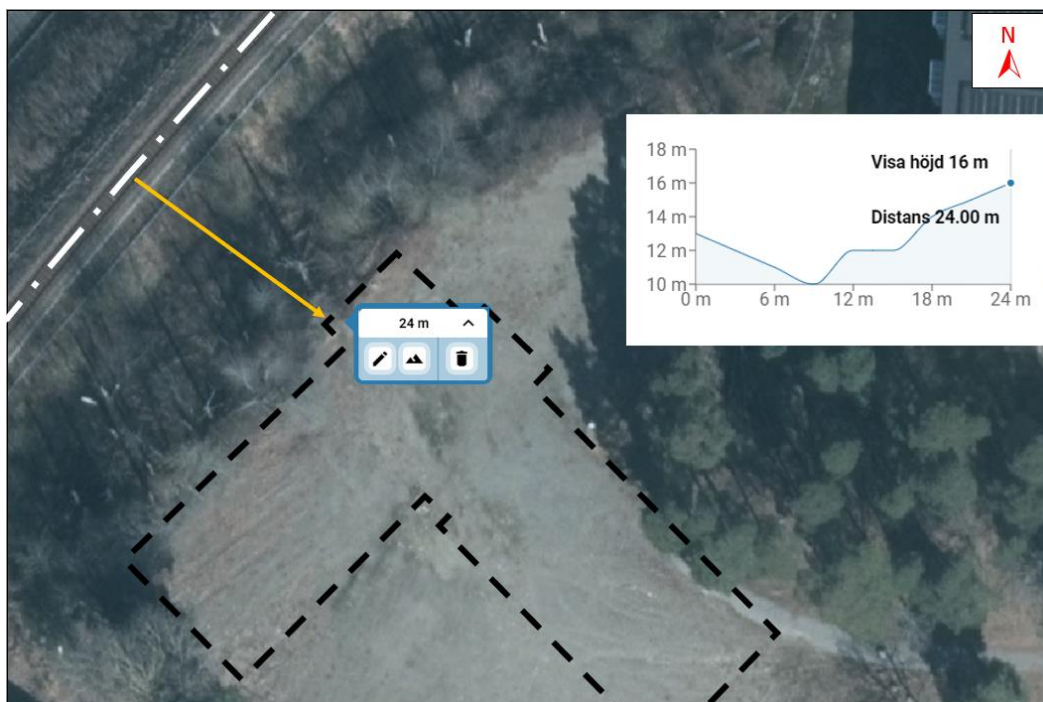
Figur 4-2. Planerad bebyggelse visas ungefärligt i svart streckad linje och intilliggande järnväg visas i vit streckad linje. Höjdskillnader visas i diagrammet i bilden, från 0 – 24 meter från järnvägen.
