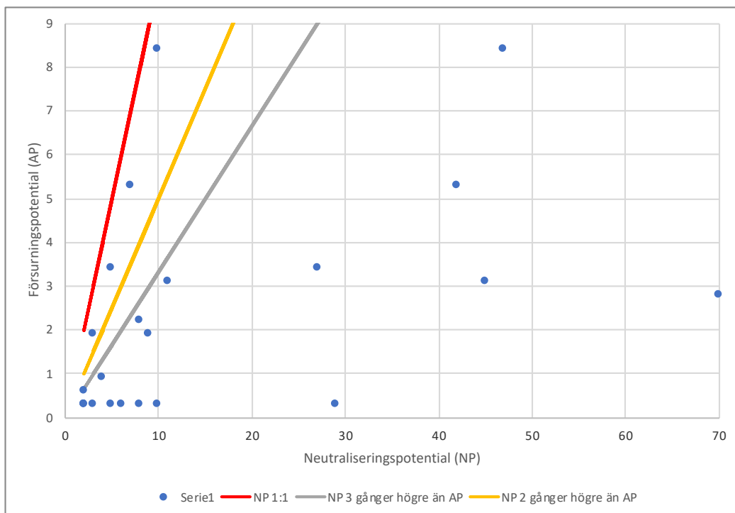
Figur 5. De analyserade provernas försurningsförmåga (AP) kontra neutraliseringsförmåga (NP). Den röda innebär att bergarternas förmåga att neutralisera är lika stor som förmågan att försura. Gula linjen visar gränsen där NP hos en bergart är två gånger högre än AP. Grå linje visar gränsen där NP är tre gånger högre än AP.
