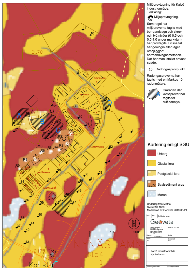
Figur 2. SGU:s jordartskarta över undersökningsområdet Kalvö industriområde. I samma karta finns även provtagningspunkter för miljöprover, radongasmätning och områden där krossprover tagits för sulfidanalys.
