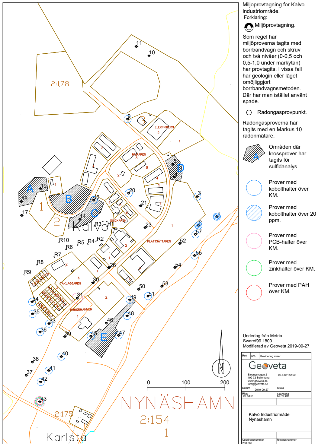
Figur 4. Punkter i undersökningsområdet där analysresultat visat på något högre värden än riktvärden för KM av kobolt, zink, PCB och PAH. För tydlighetens skull har prover där värden på kobolt överstiger 20 ppm markerats speciellt, då detta värde ligger mellan KM och MKM. Nummerade punkter motsvarar figur 3 och visar punkter för miljöprover, radongasprovpunkt och områden för krossprover för sulfidanalys.
